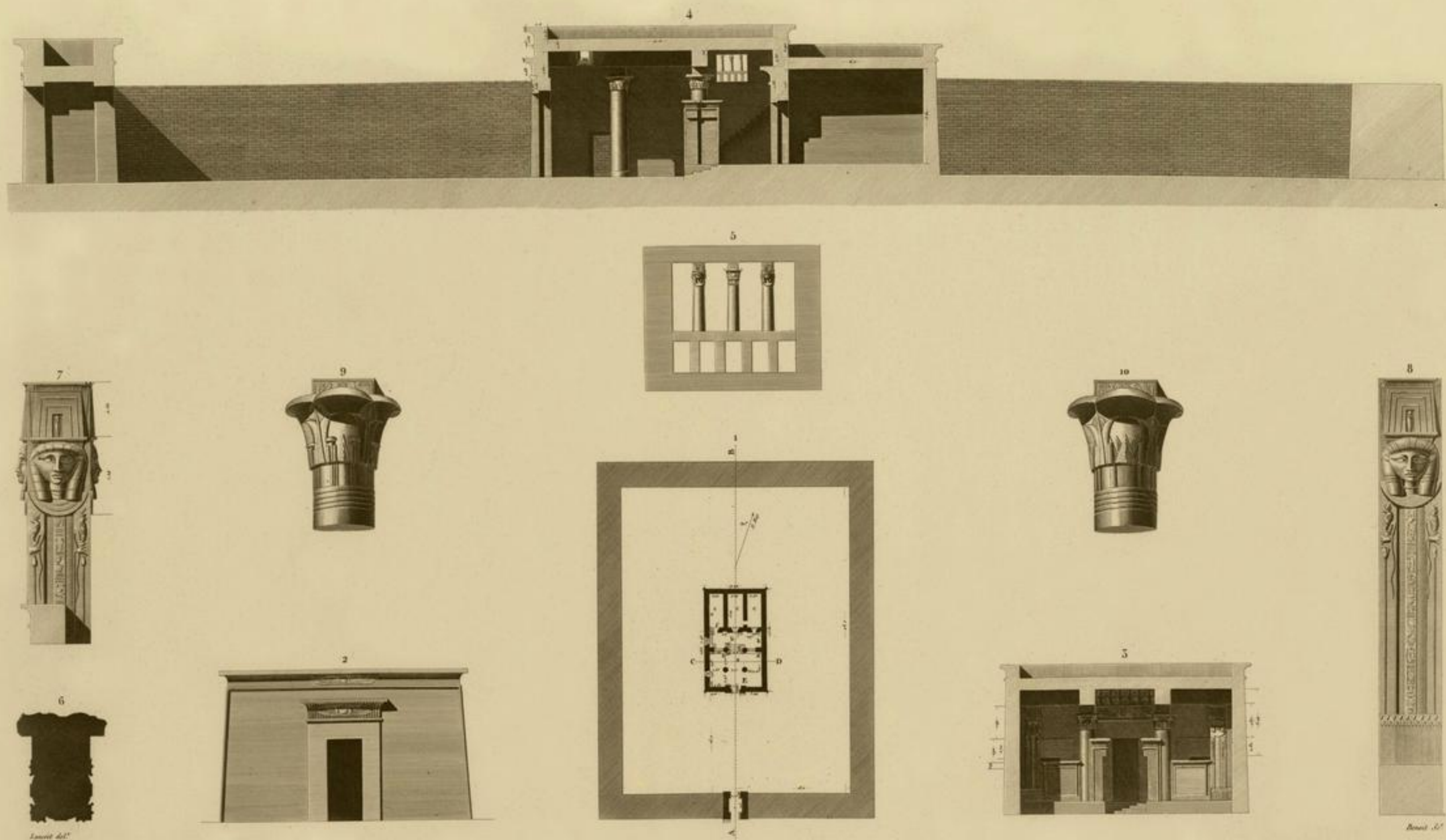
PLAN, ÉLEVATION, COUPES ET DÉTAILS DE CHAPITEAUX ET DE PILASTRE DU TEMPLE DE L'OUEST.
