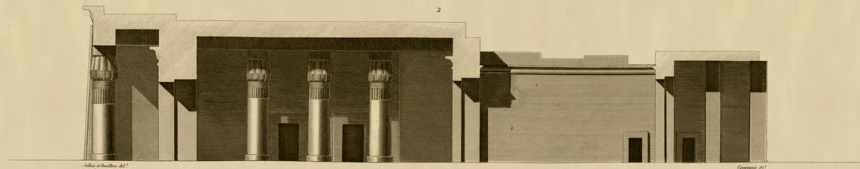
ÉLEVATION ET COUPE LONGITUDINALE DU PALAIS.
