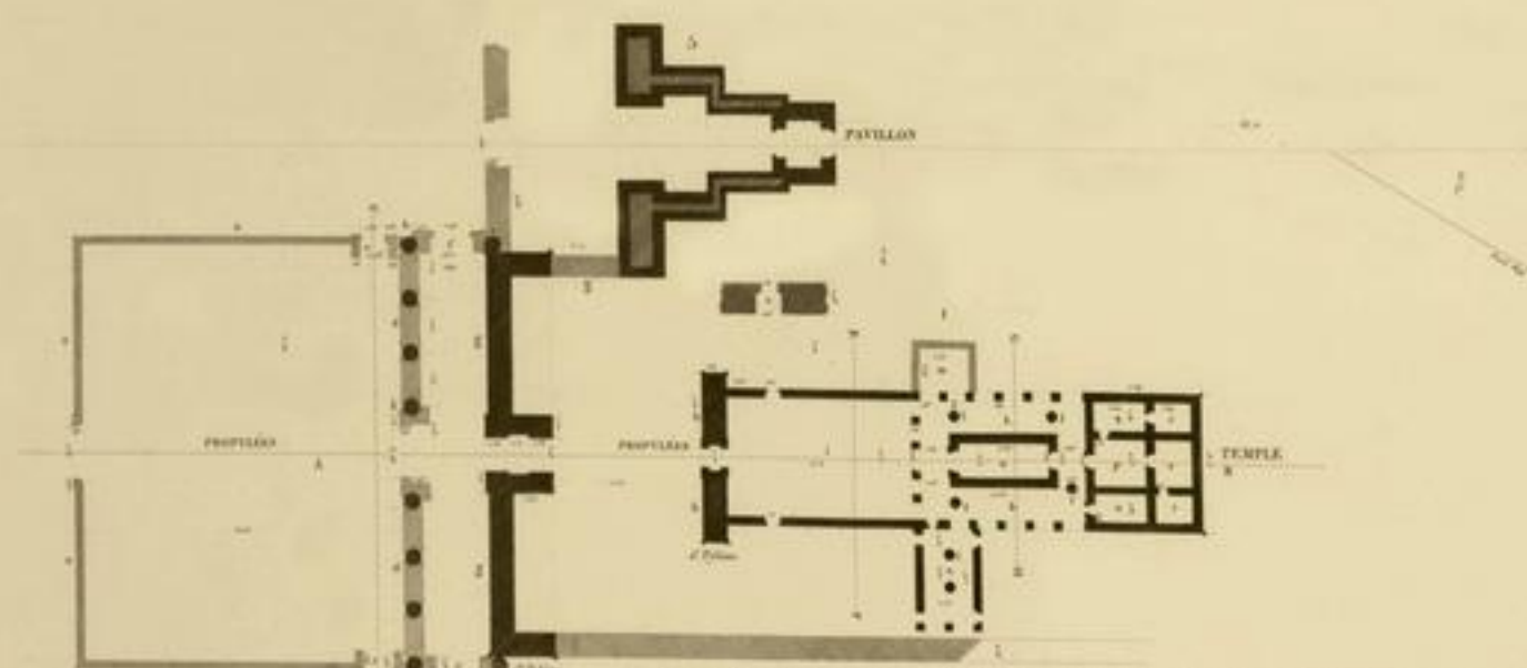
1.4 PLAN ET COUPE LONGITUDINALE DU TEMPLE ET DE SES PROPYLEES.
