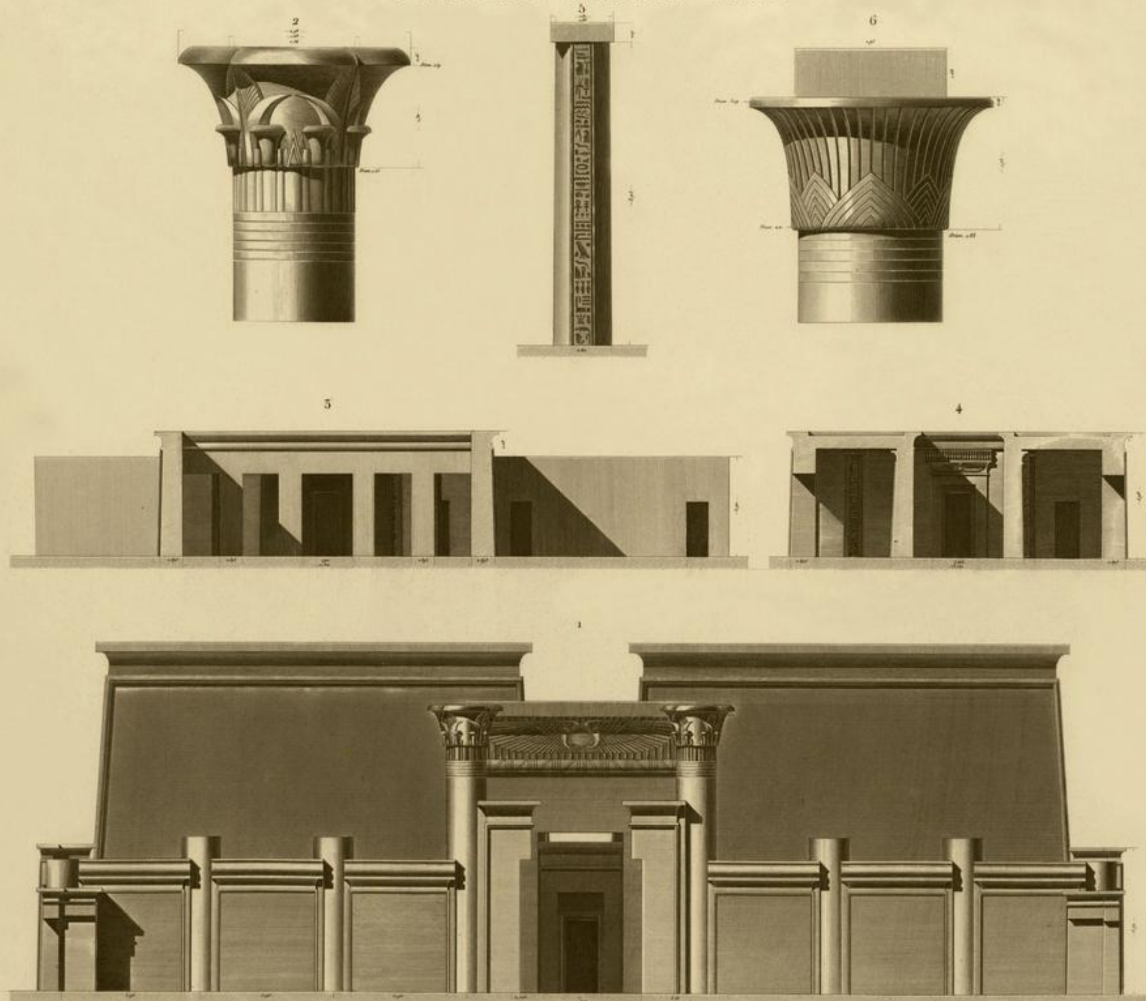
1.25.4.5 ÉLEVATION ET CHAPITEAU DES PROPYLÉES, COUPES TRANSVERSALES ET DÉTAIL D'UNE COLONNE DU TEMPLE. 6 DÉTAIL DU CHAPITEAU DES COLONNES DE LA COUR DU PALAIS.
