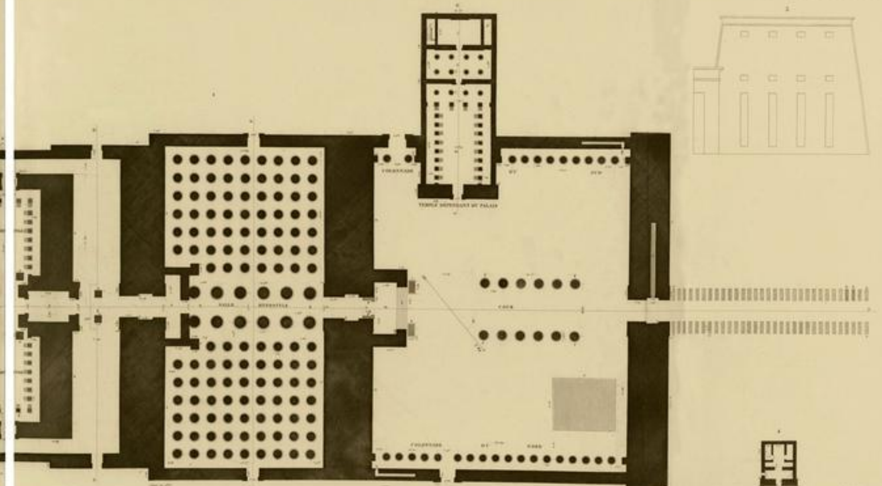
1. PLAN, COUPE GÉNÉRALE ET ÉLEVATION DU PALAIS. 2. PLAN D'UN PETIT TEMPLE PRÈS DE L'ENCRISTE DU PALAIS.
