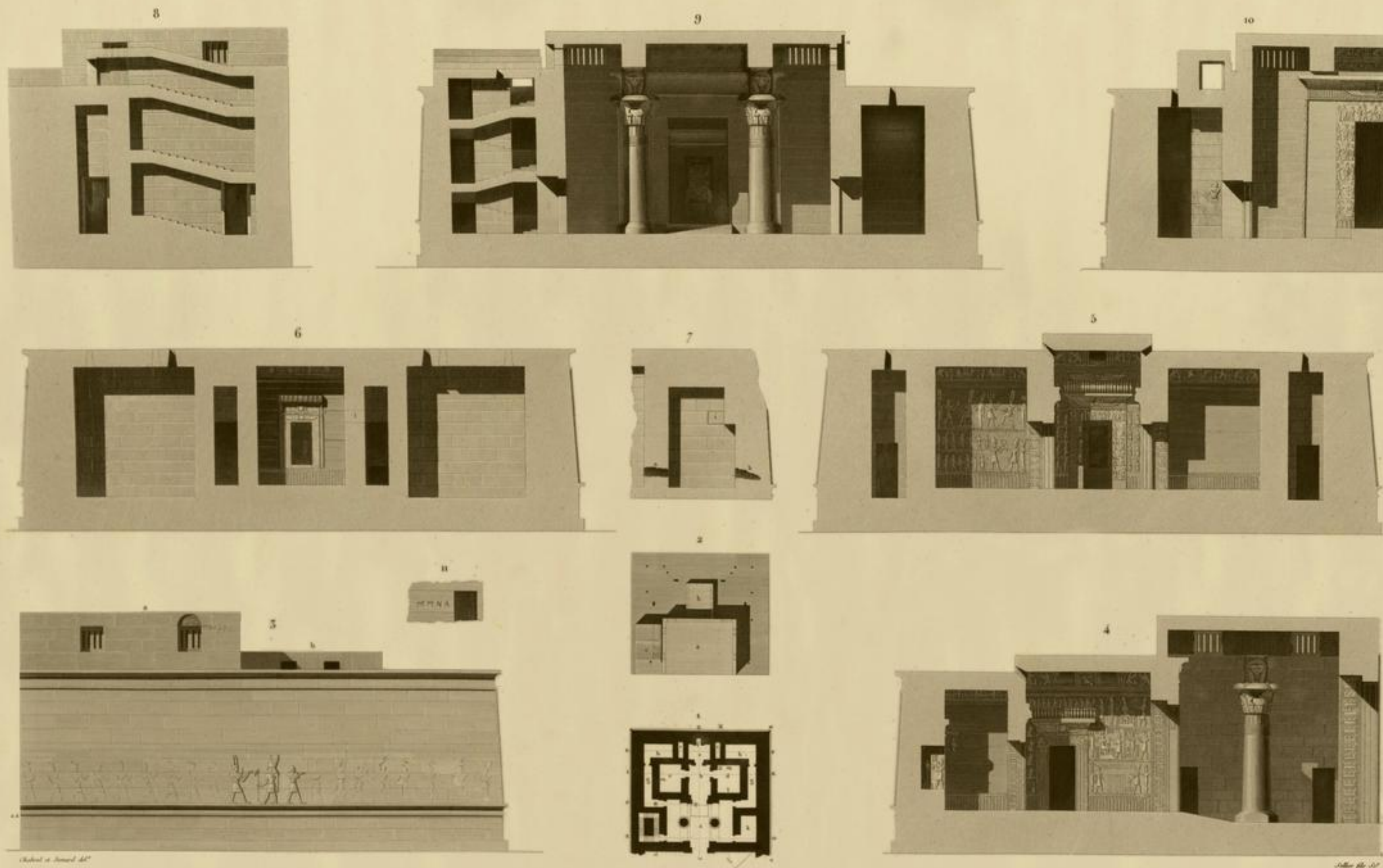
PLANS ÉLEVATION COUPES ET DÉTAILS DU PETIT TEMPLE DU SUD.
