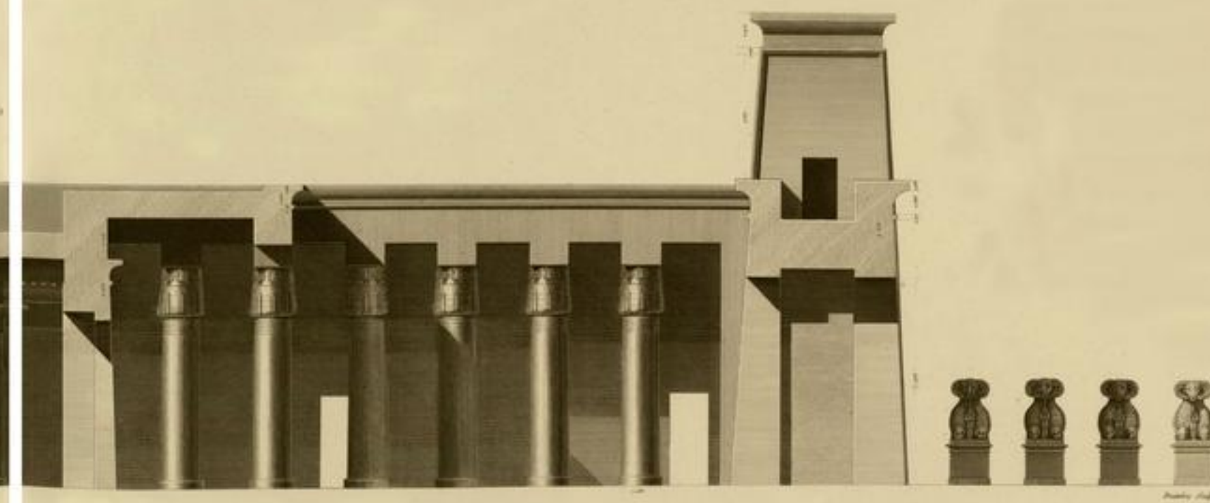
1, 2, 5 COUPES LONGITUDINALES ET TRANSVERSALES. 3, 4, 6 DÉTAILS DE CHAPITEAUX DU GRAND TEMPLE DU SUD.
