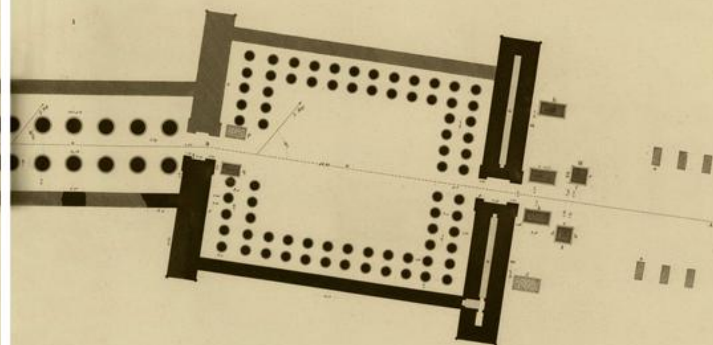
PLAN ET COUPE LONGITUDINALE DU PALAIS .
