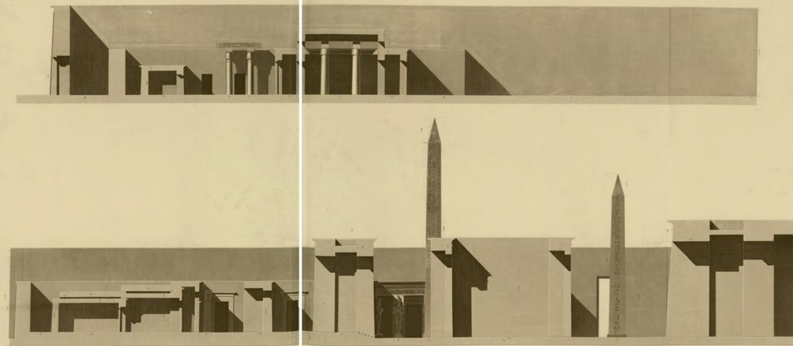
TROISIEME ET QUATRIEME PARTIES DE LA COUPE LONGITUDINALE DU PALAIS.
