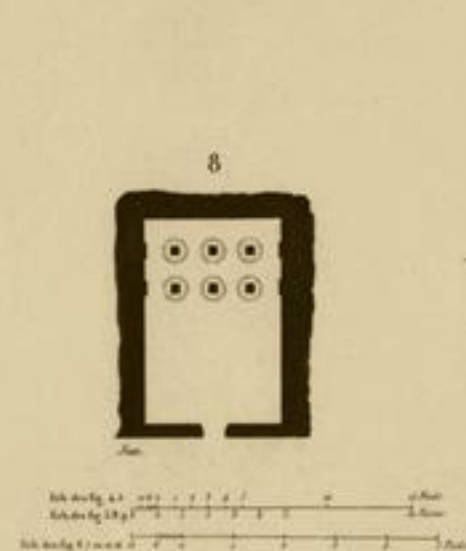
1. 2 VUES DES HYPOGÉES. 5...7 PLAN, COUPES ET DÉTAILS DE L'HYPOGÉE PRINCIPAL. 8...14 PLANS, DÉTAILS ET PEINTURES DE DIVERS HYPOGÉES.
