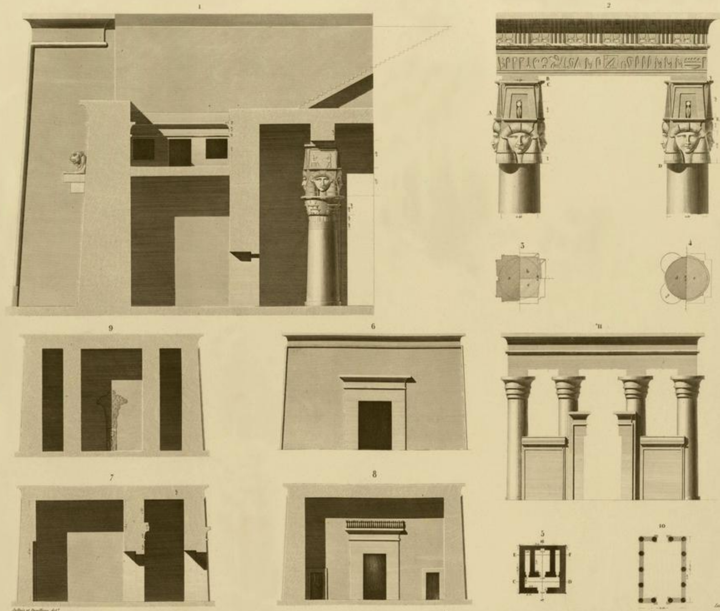
1 COUPE DU 2 e PORTIQUE DU GRAND TEMPLE. 2. 5. 4 DÉTAILS DU PETIT ÉDIFICE DE LA TERRASSE. 5. 9 PLAN, ÉLEVATION ET COUPES DE L'ÉDIFICE DU SUD. 10. 11 PLAN ET ÉLEVATION DE L'ÉDIFICE DU NORD.
