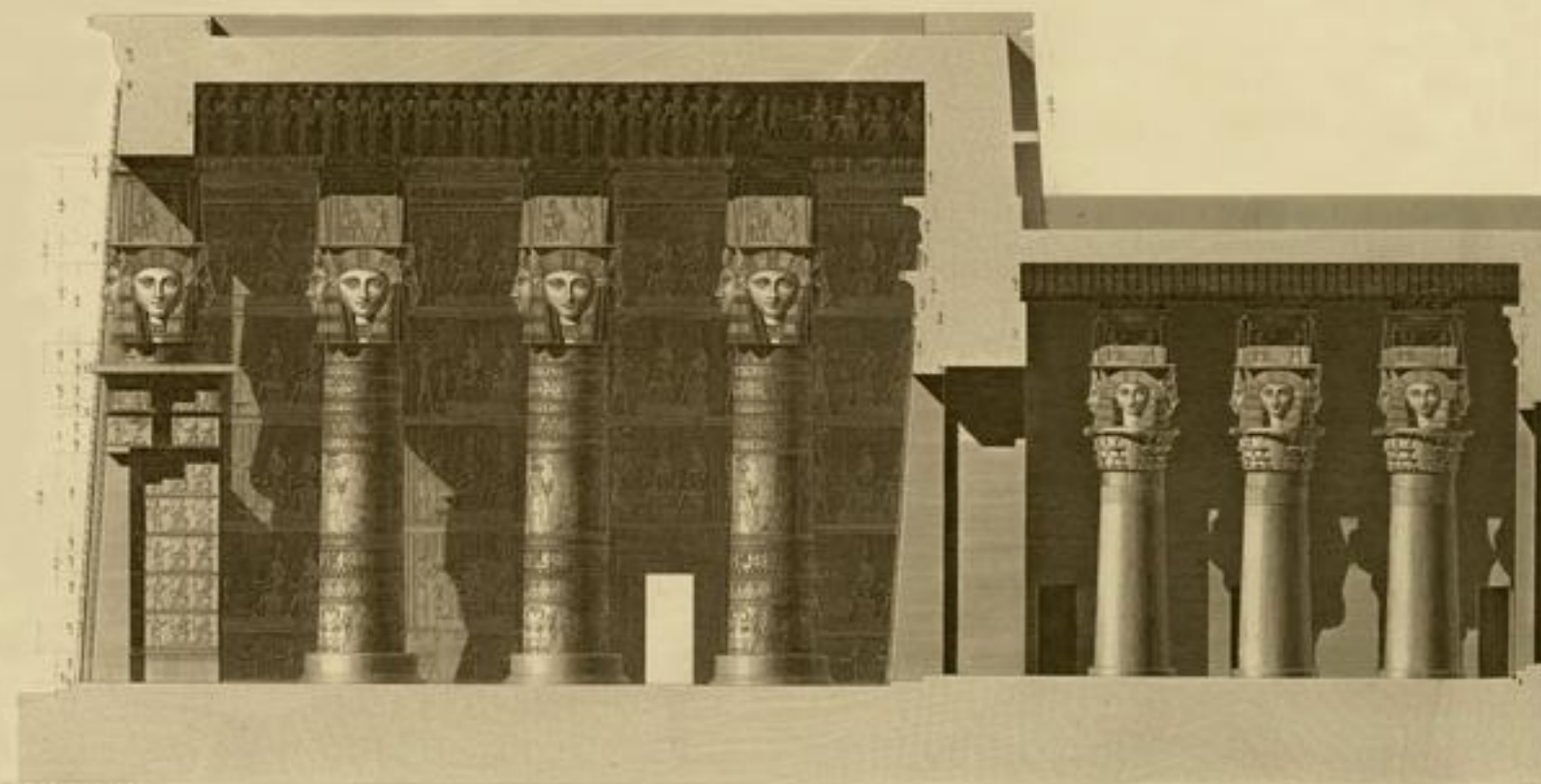
ÉLEVATION LATÉRALE ET COÛPE
