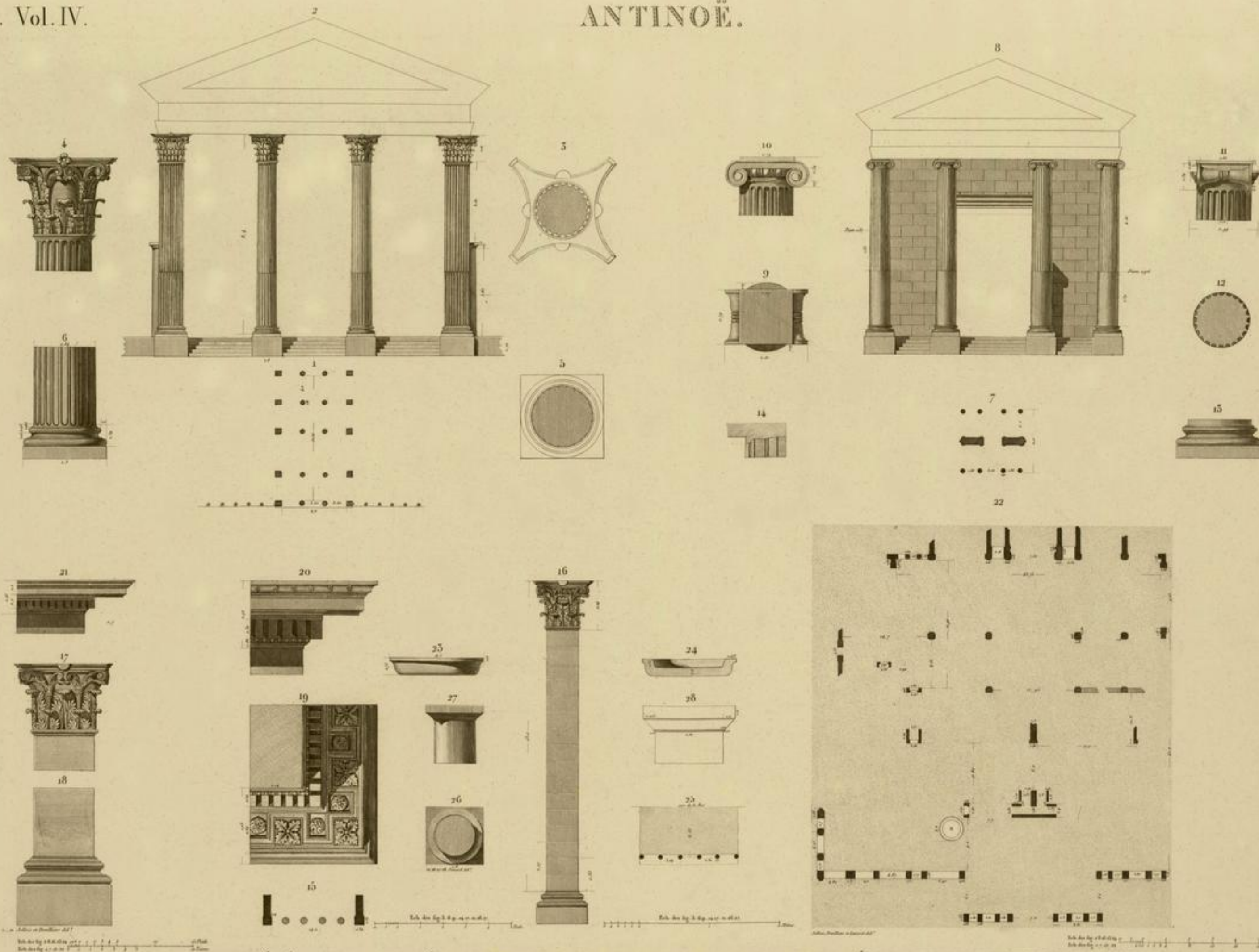
1...20 PLANS, ÉLEVATIONS ET DÉTAILS DE DIVERS PORTIQUES. 21...24 PLAN ET DÉTAIL D'UN BATIMENT DE BAINS. 25...28 COLONNADE DE LA RUE PRINCIPALE.
