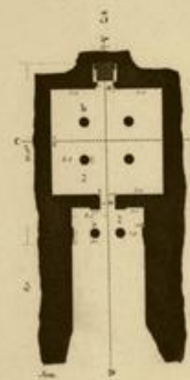
1. 2 VUES DES HYPOGÉES. 5...7 PLAN, COUPES ET DÉTAILS DE L'HYPOGÉE PRINCIPAL. 8...14 PLANS, DÉTAILS ET PEINTURES DE DIVERS HYPOGÉES.
