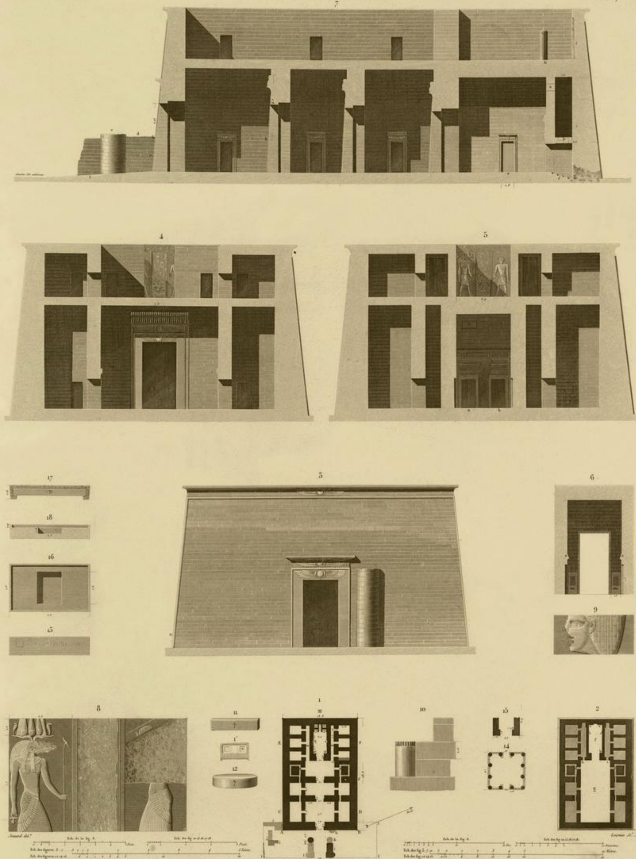
1.....15 PLANS, ÉLEVATION, COUPES ET DÉTAILS D'UN TEMPLE ÉGYPTIEN, SITUÉ VERS L'EXTREMITÉ OCCIDENTALE DU LAC APPELÉ BIRKET EL QEROUN. 14...18 PLANS ET DÉTAILS DE PLUSIEURS ANTIQUITÉS DES ENVIRONS.
