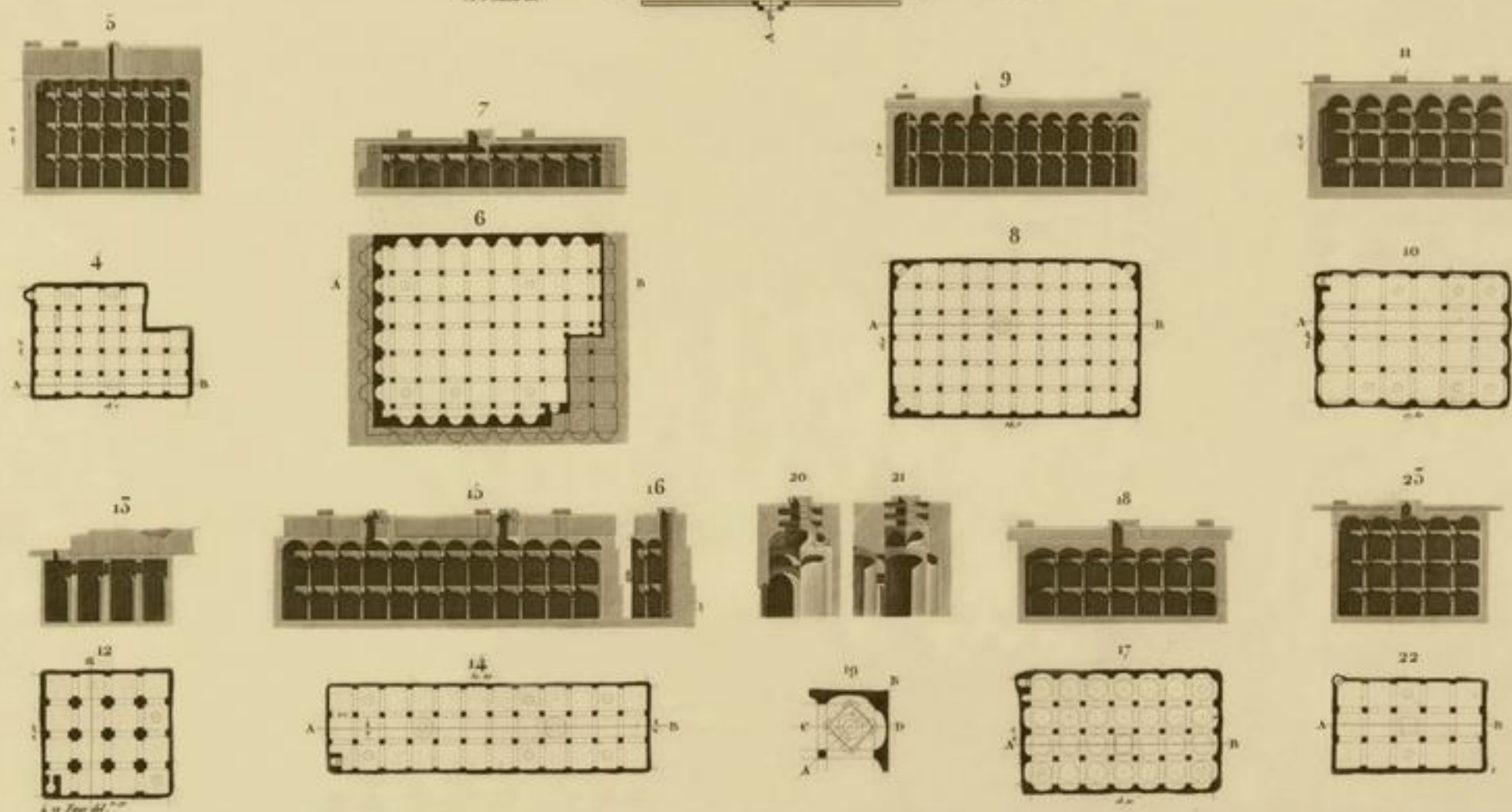
1. 2. 3. PLAN, ÉLÉVATION ET COUPE D'UNE ANCIENNE ÉGLISE DITE MOSQUÉE DES MILLE COLONNES OU DES SEPTANTE. 4...25 PLANS, COUPES ET DÉTAILS DE HUIT DES PRINCIPALES CITERNES DE L'ANCIENNE VILLE.
