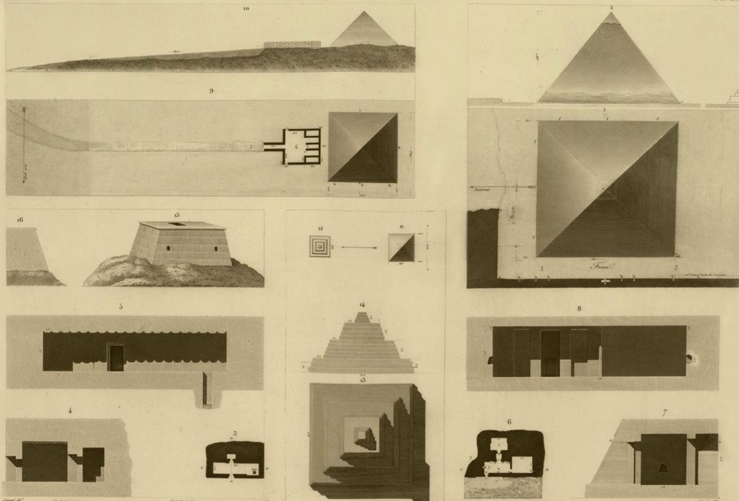
1. 8 PLAN ET ELEVATION DE LA 2 e PYRAMIDE, PLANS ET COUPES D'UN HYPOGÉE À L'OUEST ET D'UN AUTRE À L'EST. 9. 10 PLAN ET ELEVATION DE LA 3 e PYRAMIDE, DE L'ÉDIFICE DE L'EST ET D'UNE GRANDE CHAUSSÉE. 11. 14 PLANS ET ÉLEVATION DE LA 4 e PYRAMIDE ET D'UNE PYRAMIDE À DÉGRÉS. 15. 16 TOMBEAU PYRAMIDAL À L'OUEST DE LA GRANDE PYRAMIDE.
