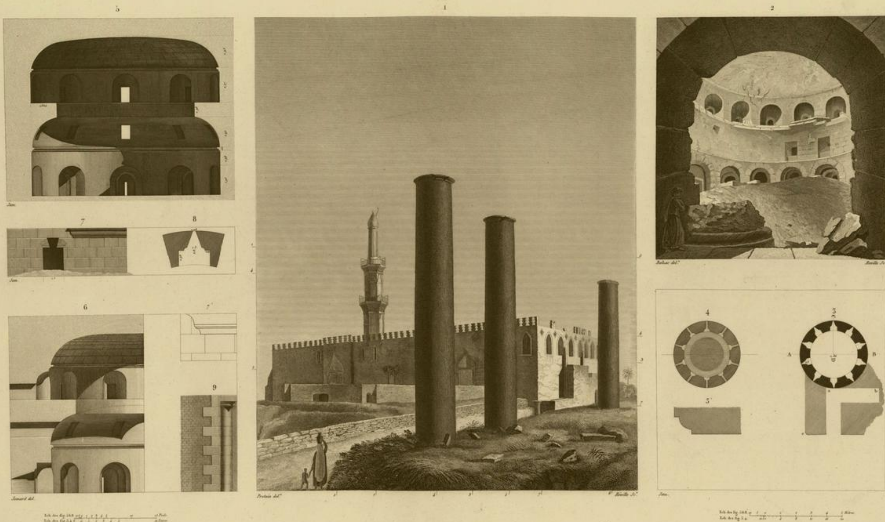
1 VUE DE TROIS COLONNES EN GRANIT, SITUÉES AU SUD DE L'ANCIENNE BASILIQUE VULGAIREMENT NOMMÉE MOSQUÉE DE S t ATHANASE. 2....9 VUE INTÉRIEURE, PLANS, COUPES ET DÉTAILS D'UNE TOUR ANTIQUE, PLACÉE AU NORD DES DEUX OBÉLISQUES, ET CONNUE SOUS LE NOM DE TOUR DES ROMAINS.
