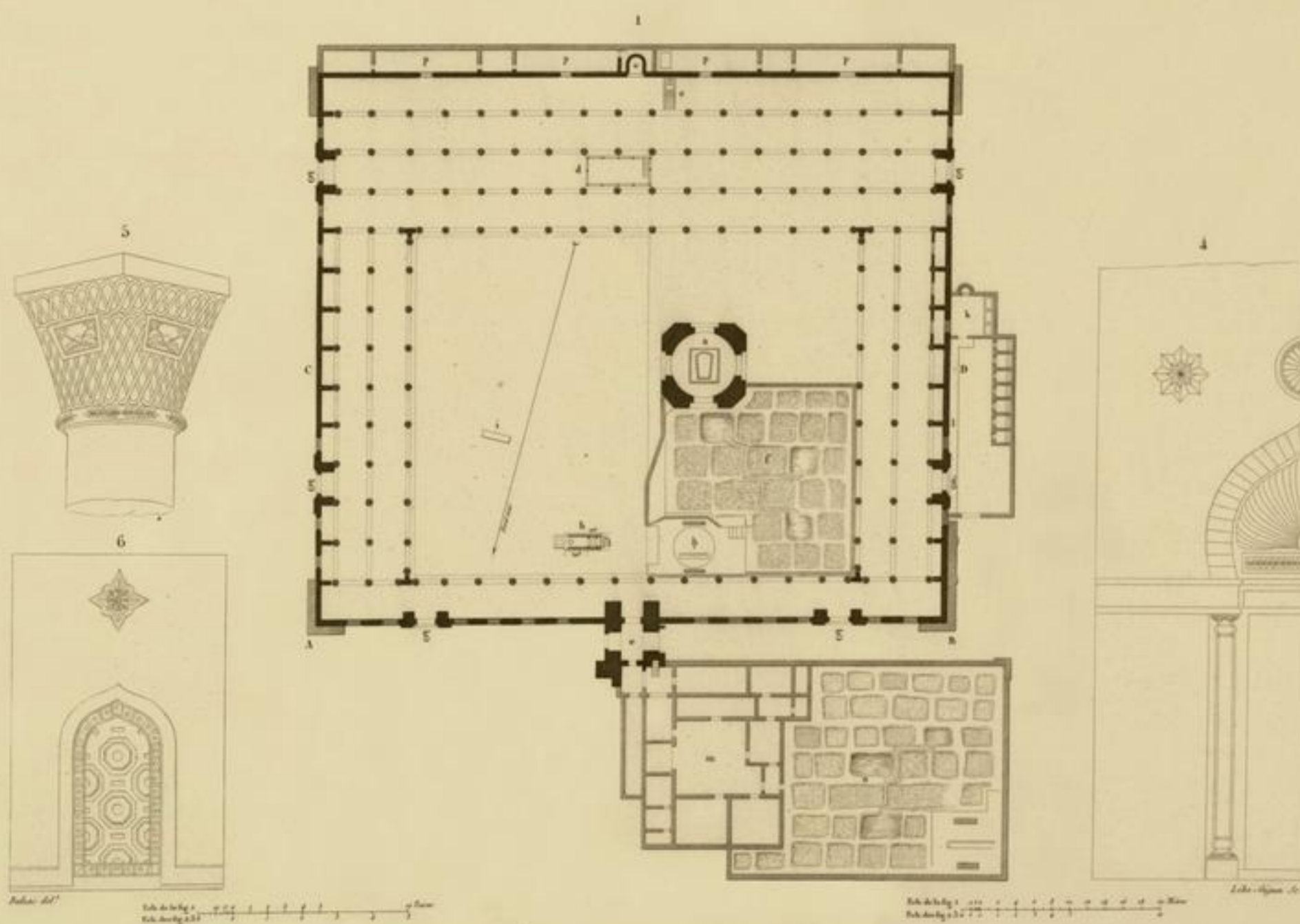
PLAN, ÉLEVATION, COUPE ET DÉTAILS D'UNE ANCIENNE BASILIQUE, VULGAIREMENT NOMMÉE MOSQUÉE DE S t ATHANASE.
