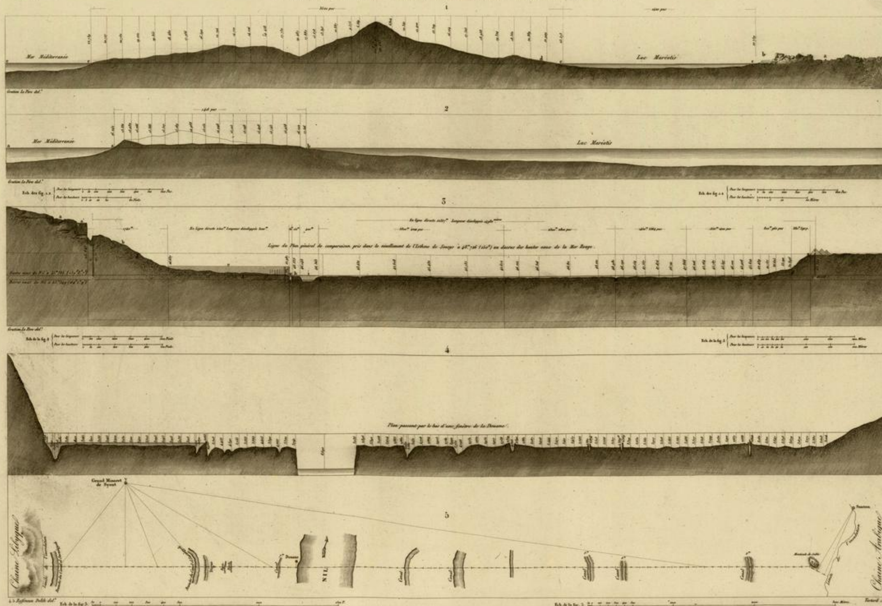
1.2 PROFILS DE NIVELLEMENT DU LAC MARÉOTIS À LA MER. 5 PROFIL DE LA VALLÉE DU NIL À LA HAUTEUR DES PYRAMIDES.
