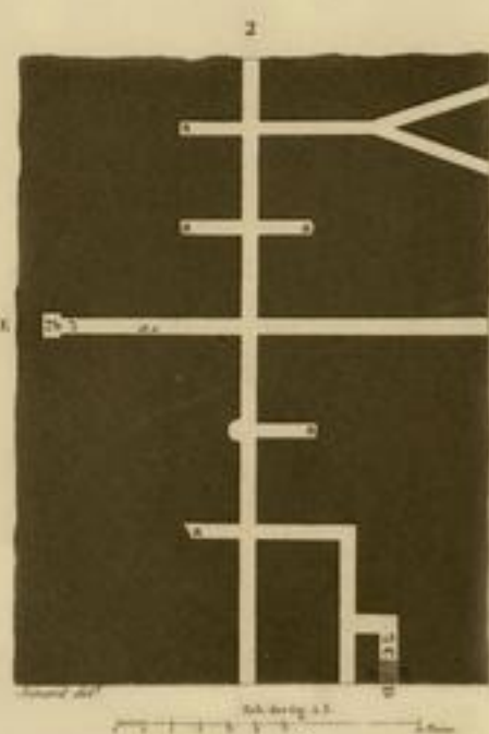
1 POIGNET D'UN COLOSSE À MEMPHIS. 2...7 PLAN, COUPE ET DÉTAILS D'UN TOMBEAU DE MOMIES D'OISEAUX À SAQQÀRAH. 8 VUE DES CARRIÈRES DE TORRAH. 9 VUE D'UN MUR ANTIQUE.
