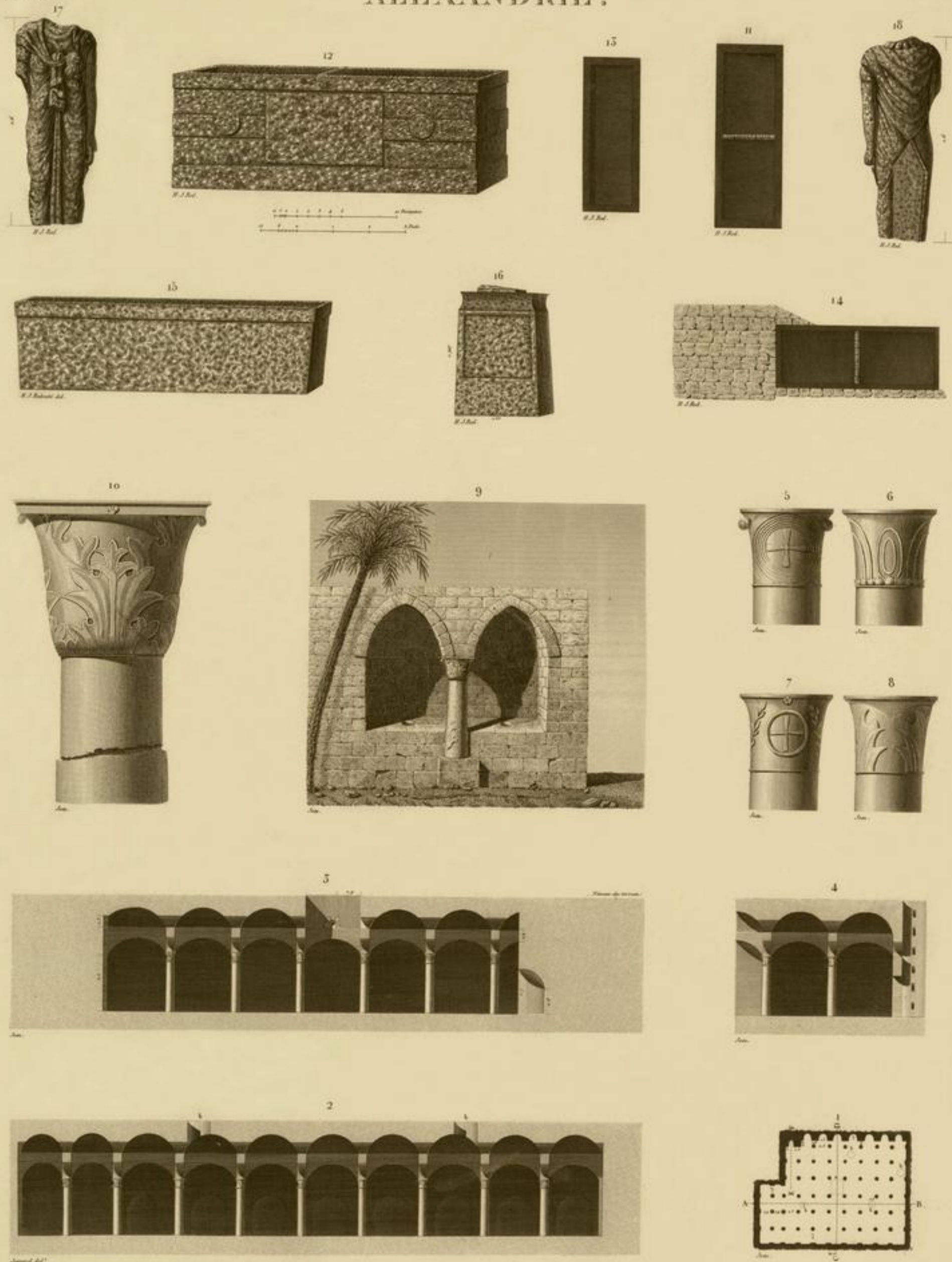
1-8 PLAN, COUPES ET DÉTAILS D'UNE GRANDE CITERNE. 9-10 DÉTAILS D'UNE COLONNE AVEC UN CHAPITEAU EN MARBRE 11-18 SARCOPHAGES, STATUE ET SOCLE EN GRANIT.
